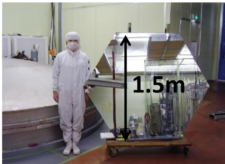
1.5mの六角形の試作鏡
